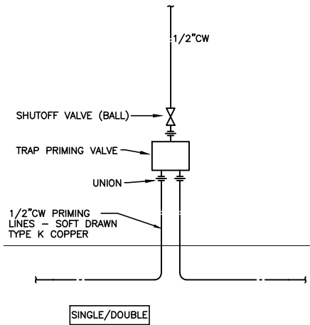
1 TRAP PRIMER DETAIL NO SCALE
