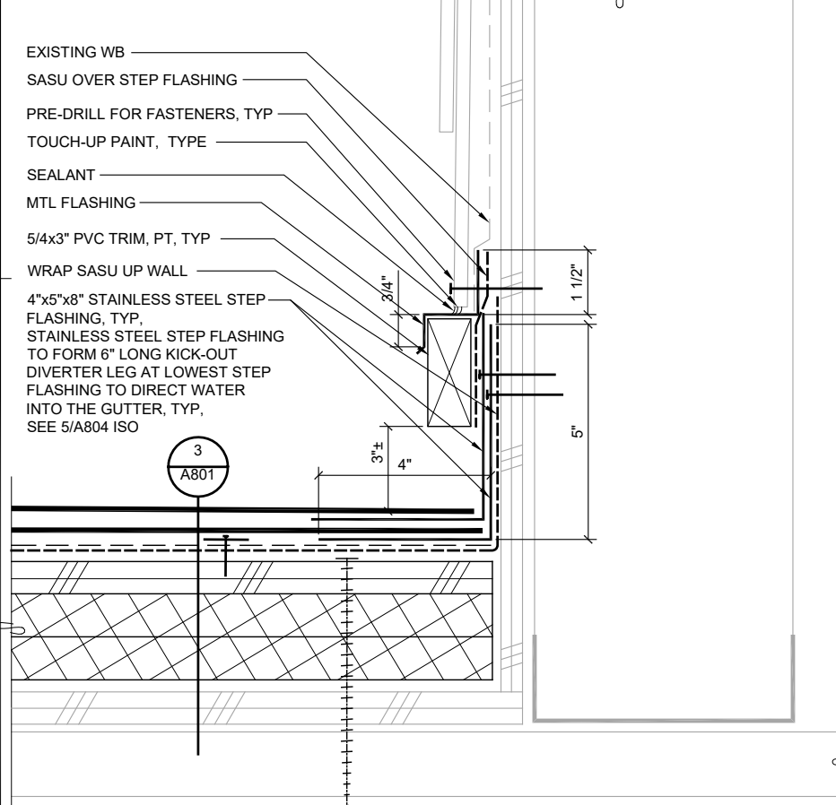
4 STEP FLASHING 21037 - X_A802-4 SCALE: 0 3\"/>
