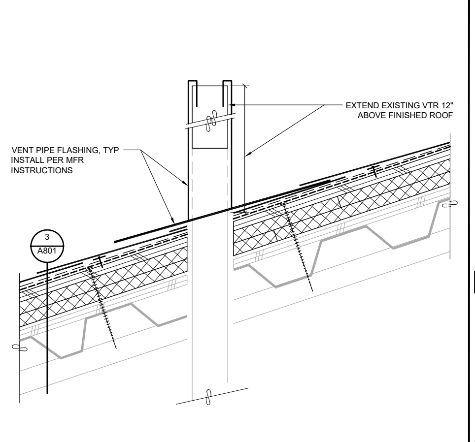
6 DEMO VTR FLASHING 21037 - X_A802-6 SCALE: 0 3\"/>
