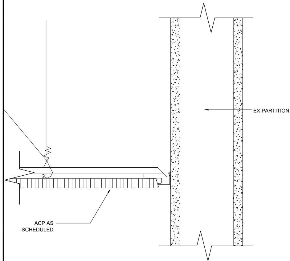
1 ACP @ WALL TYP 20014/A901-1 SCALE: 0 3" 6"
